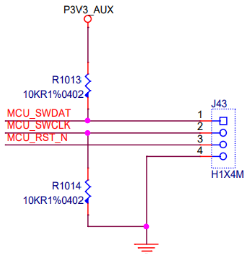
图 2-17 MCU Header
