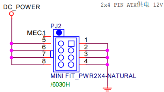
图 2-5 主板电源接口定义
